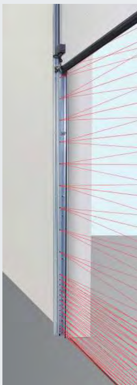
Lichtgitter HLG in der Zarge integriert
