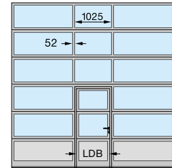
ALR F42, ALR F42 Thermo, ALR 67 Thermo Schlüpftüranordnung Mitte
